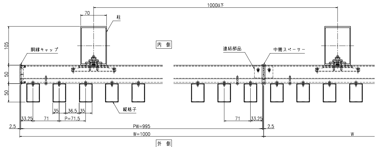
横断面詳細図 (S=1/3)
